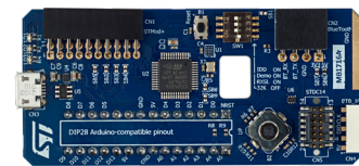
STM32C0316-DK 小型評価ボード
